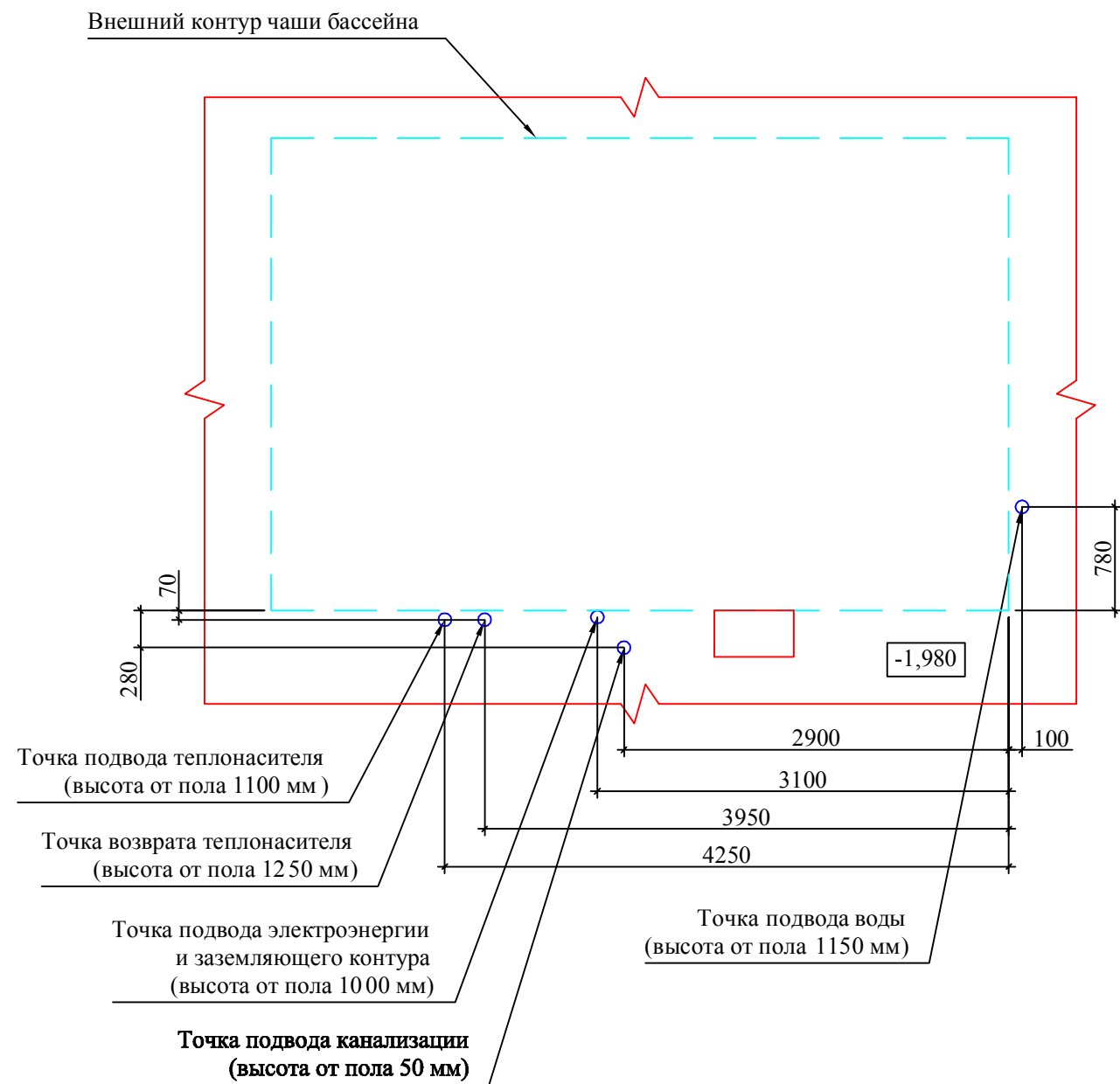
Схема 1. Размещение точек подвода коммуникаций
